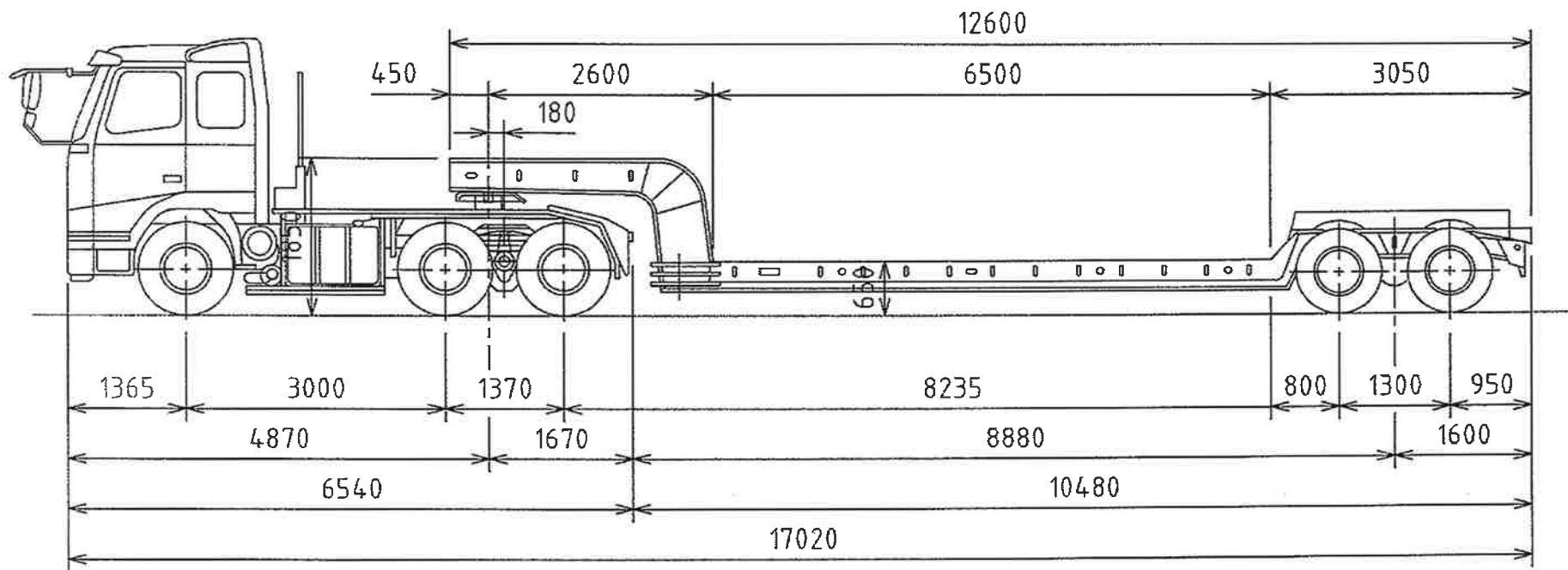
(ボルボFH16Z型(6x4)トラクタ)
